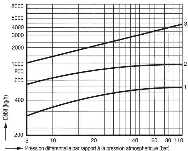
Diagramme de débit PN160
