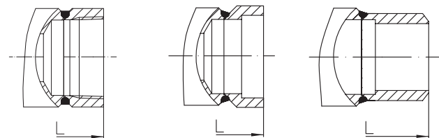
Fig. 600/601...2 à manchons taraudés
