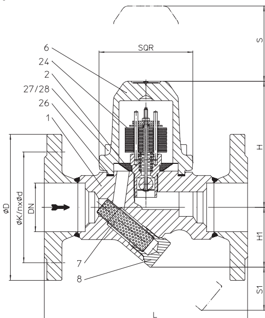
Fig. 601...1 à brides
